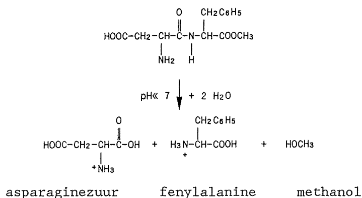
figuur 3 De zure hydrolyse van Aspartaam
